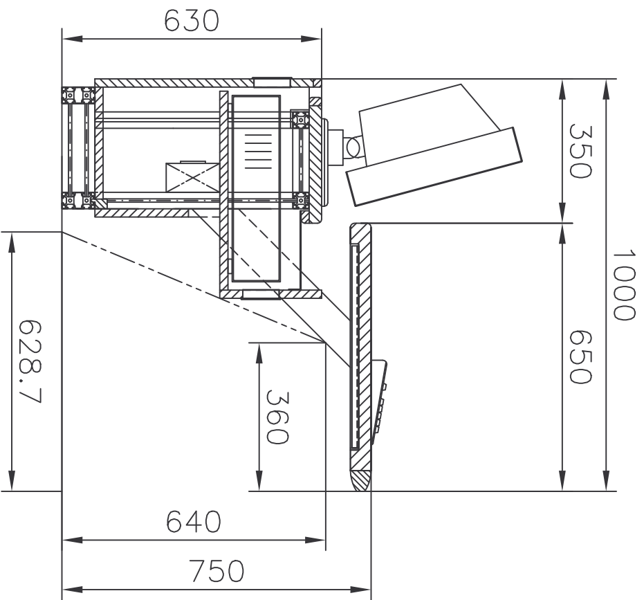
Pultquerschnitt mit 20"-Flachmonitor
