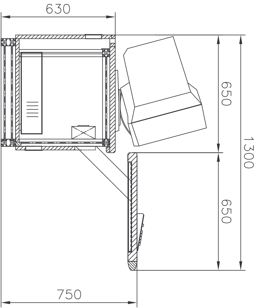
Pultquerschnitt mit 21"-Monitor
